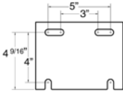
Mounting Plate (GBA-642, GBA-542)
