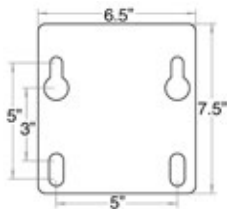
Mounting Plate (GBA-180)
