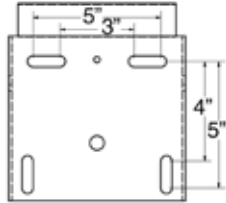
Mounting Plate (GBA-648, GBA-548)
